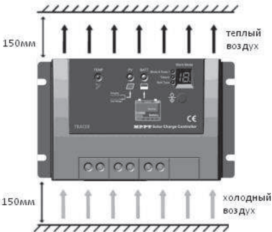
Рис.2. Установка контроллера
