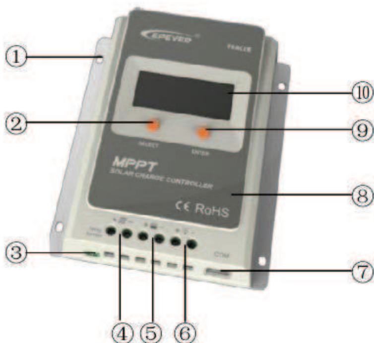
Рис.1. Органы управления и индикации контроллера
