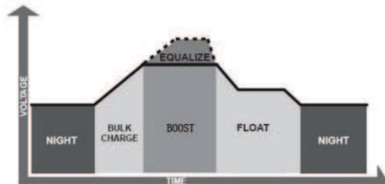
Рис.5. Стадии заряда аккумулятора
